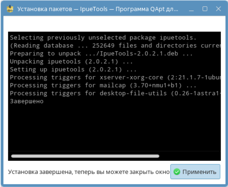
Рисунок 8 – Окно «Установка пакетов» по завершению установки
