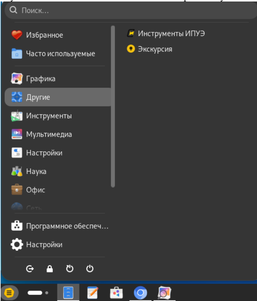
Рисунок 5 – Меню приложений
